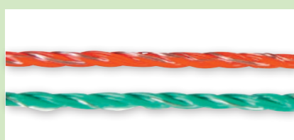
alle Leiter = gute Leitfähigkeit durch 3 x 0,20 mm Edelstahlleiter
